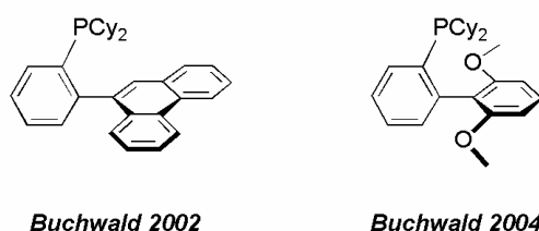
Abbildung 22. Buchwalds Weiterentwicklungen für die Kreuzkupplung von 2,6-substituierten Arylbromiden mit 2,6-substituierten Arylboronsäuren.
