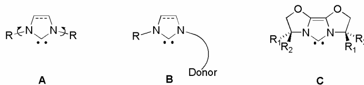
Abbildung 5. Ligandenkonzepte.
