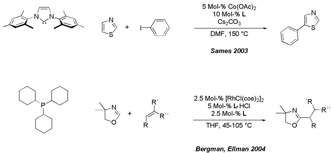
Schema 5. C-H-Aktivierung mit Hilfe von phosphin- und carbengestützten Katalysatoren.
