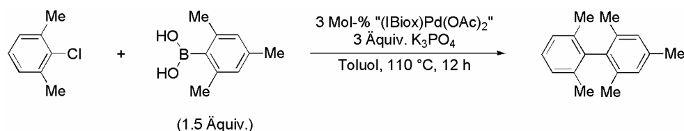
Schema 23. Testreaktion für das Ligandenscreening.
