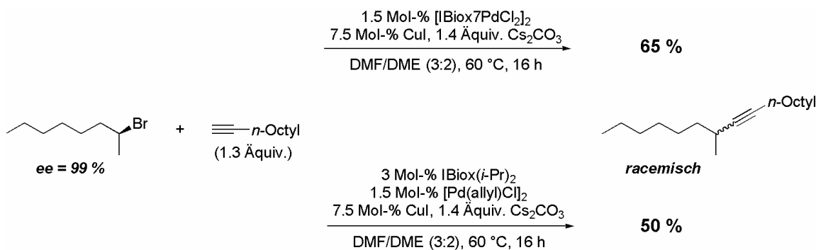
Schema 36. Versuche zur enantioselektiven Alkyl-Sonogashira-Reaktion.
