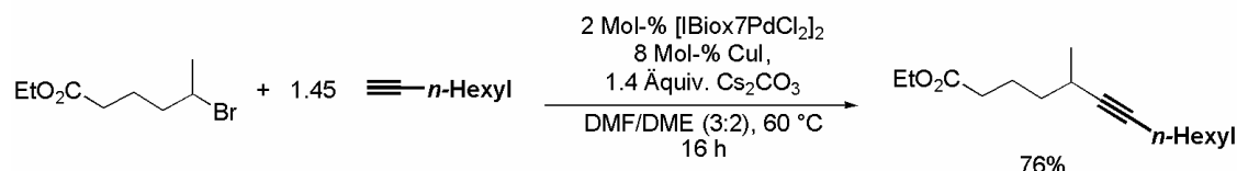
Schema 42. Sonogashira-Reaktion mit sekundären Alkylbromiden.
