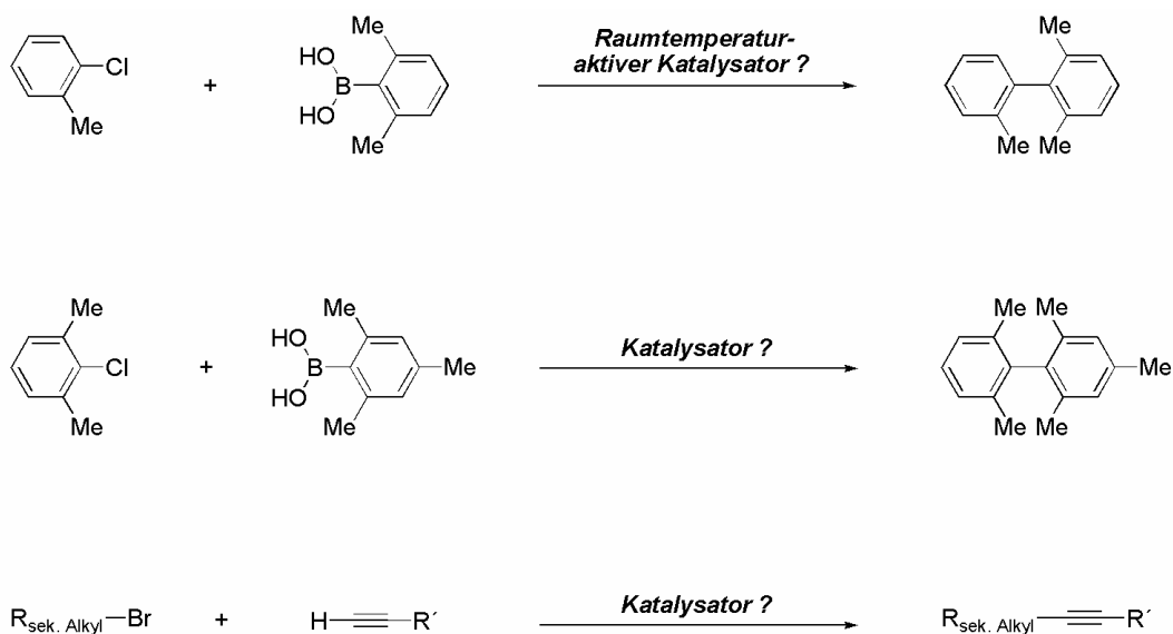
Schema 6. Ungelöste Probleme in der Kreuzkupplungsschemie.
