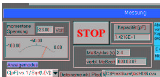
Abbildung A.13: Messbereich bei der Kapazitäts-Spannungs-Messung
