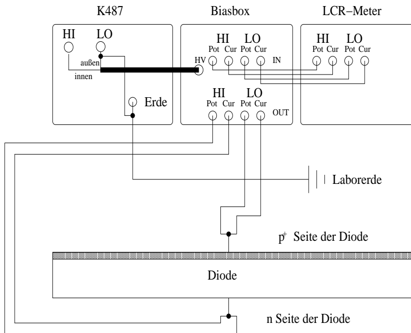
Abbildung B.6: Messaufbau für die Kapazitäts-Spannungs-Messung
