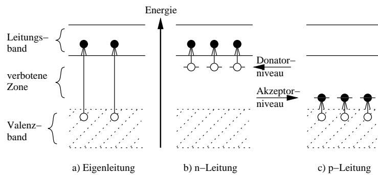
Abbildung A.2: a) Skizze der Eigenleitung bei einem Halbleiter b) Skizze der n-Leitung c) Skizze der p-Leitung bei einem Halbleiter (siehe Abschnitt A.1.2)
