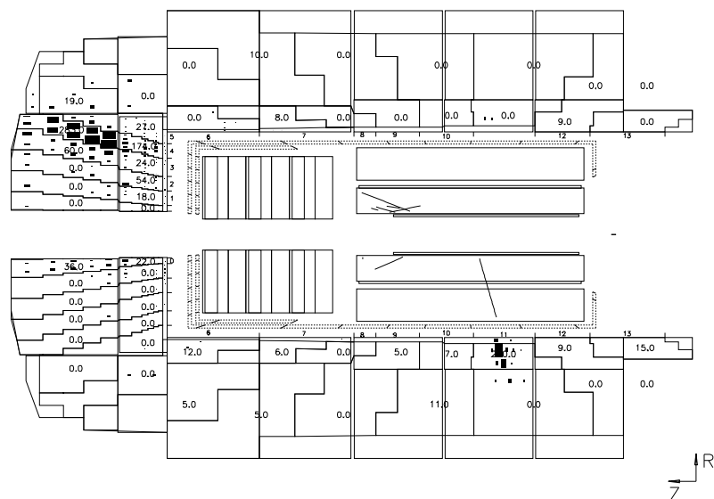
Abbildung 2.7: Geometrische Struktur der Big Tower im Flüssigargon-Kalorimeter in der r - z -Projektion [And-1993]. Kalorimeterzellen werden dergestalt zu Big Tower zusammengefasst, daß diese auf den Wechselwirkungspunkt ausgerichtet sind. Im linken oberen Teil ist die Signatur eines hadronischen, im mittleren unteren Teil eines elektromagnetischen Schauers durch ein gestreutes Elektron zu sehen.
