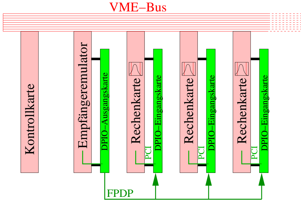
Abbildung 4.19: FTT-L3-Testaufbau zur Bestimmung von Systemkenngrößen. Da zunächst keine Empfängerkarte zu Verfügung steht, wird diese durch eine Prozessorkarte mit aufgesteckter DPIO-Ausgangskarte und entsprechender Programmierung emuliert. In die Programmierung der Kontrollkarte wurden zusätzliche Datentransfermöglichkeiten zu einem Steuerungsrechner implementiert, um Testdaten in das System ein- und Ergebnisse auslesen zu können.
