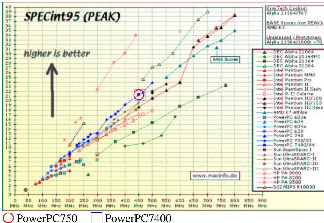
Abbildung 4.3: SPEC95-Test für verschiedene Prozessoren mit Testprogrammen, die ausschließlich Operationen mit ganzzahligen Werten ausführen [Mac-2002]. Einkreist ist der Wert für den Prozessor PowerPC 750. Der Nachfolgetyp PowerPC 7400 zeichnet sich nur durch eine Optimierung für Gleitkommaoperationen aus, so daß dieser den gleichen SPEC-Wert wie der PowerPC 750 erreicht.
