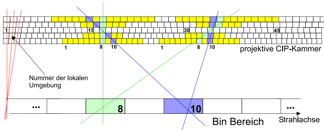
Abbildung 2.3: Schematische Ansicht der CIP2000-Kammer mit projektiv zum Wechselwirkungspunkt (Bin 10) hin ausgerichteten Pads. Aus Treffern in verschiedenen Lagen wird versucht, eine Teilchenspur in der rz -Ebene zu rekonstruieren und diese zur Strahlachse zu extrapolieren. [Urb-2000a]
