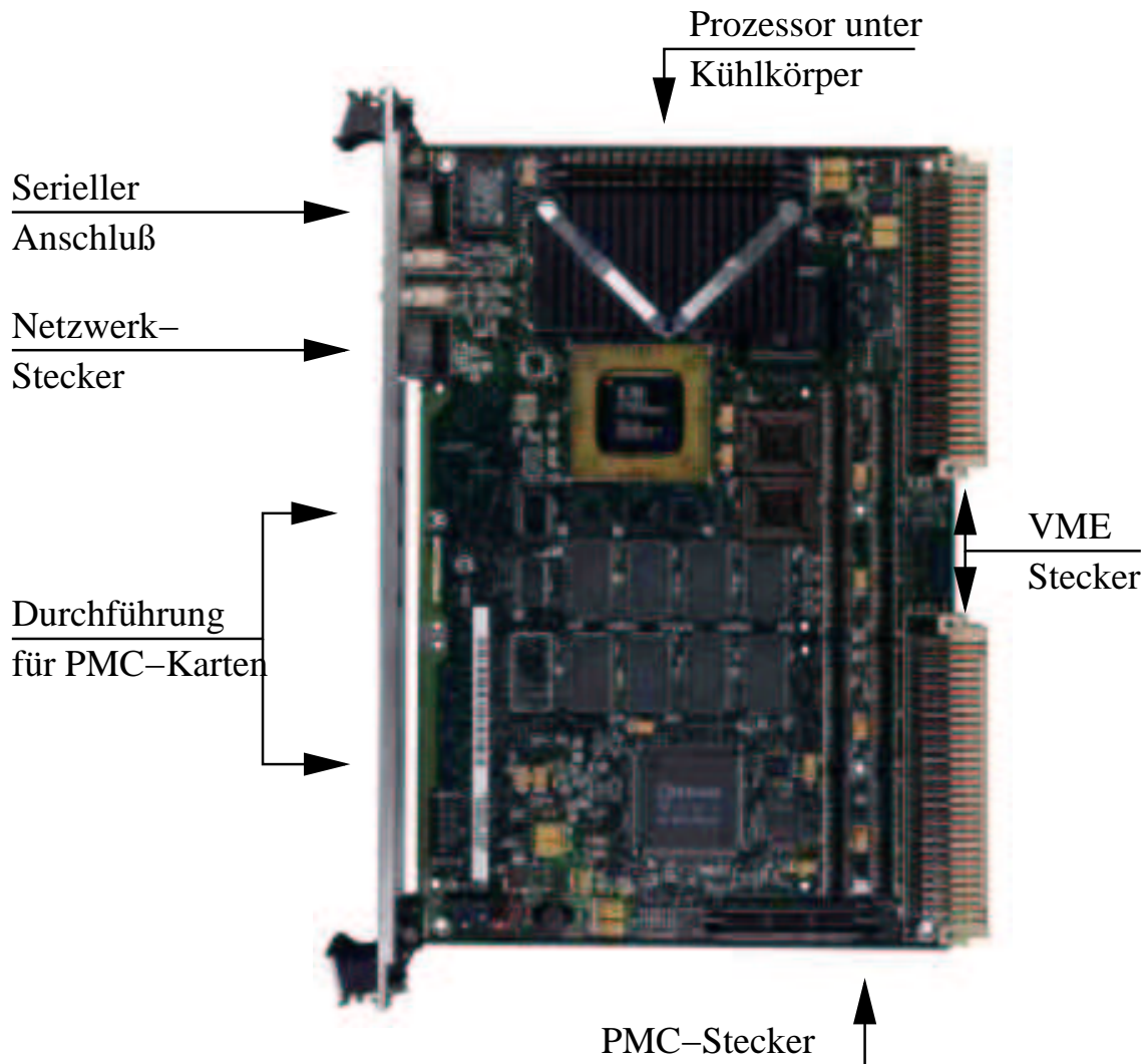
Abbildung 4.6: MVME2400-Karte von Motorola [Mot-1994]. Im oberen Teil der Karte befindet sich unter einem Kühlkörper der PowerPC 750-Prozessor, in der Mitte befinden sich die Bänke für Speicherbausteine. Für den Datentransfer zu der Karte hin oder von der weg Karte sind ein serieller Anschluß, ein Netzwerkanschluß, eine VME-Schnittstelle und zwei PMC-Steckplätze integriert.
