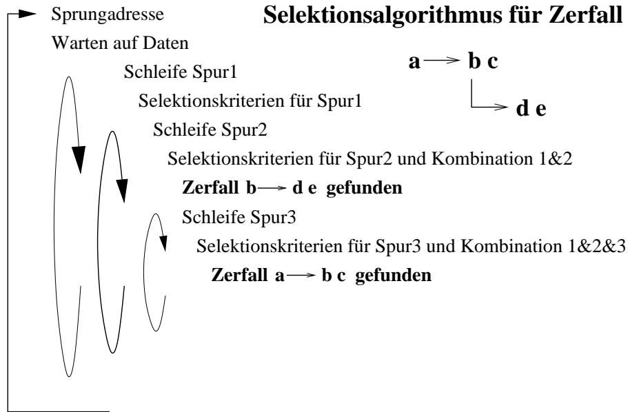
Abbildung 4.16: Schematische Darstellung eines spurbasierten Selektionsalgorithmus für FTTL3. Der Algorithmus ist generell zur Selektion eines zweistufigen Zerfalls a \rightarrow bc \rightarrow dec ausgelegt, kann aber auch durch Weglassen der innersten Schleife für die Selektion reiner Zweiteilchenzerfälle verwendet werden. Beispiele für Selektionskriterien in den einzelnen Schleifen sind im Text gegeben.
