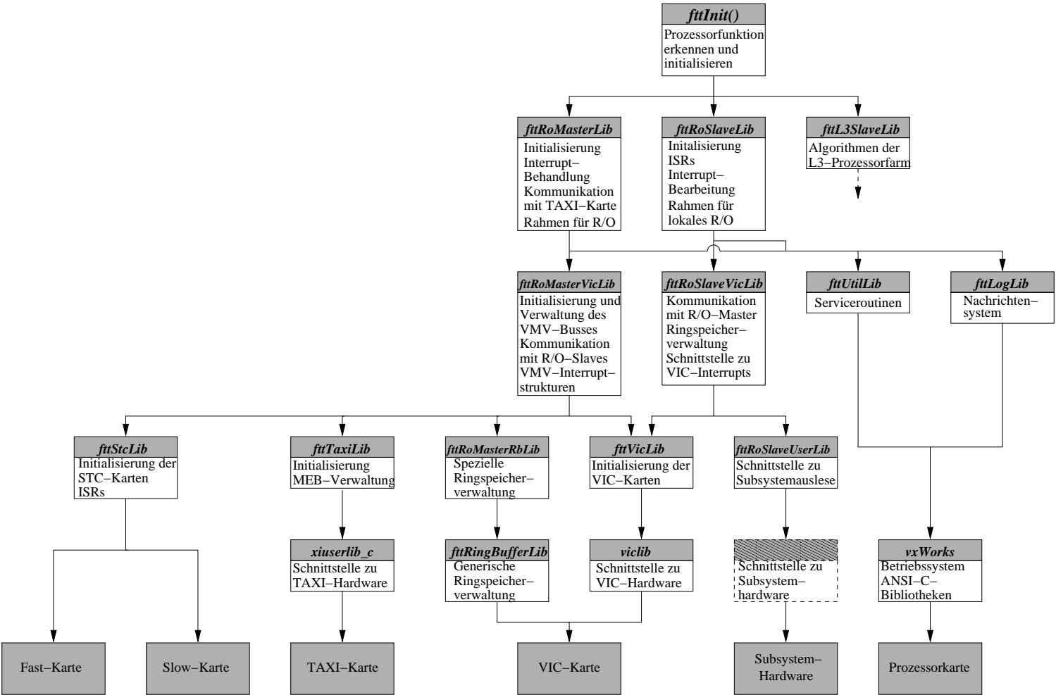
Abbildung A.4: Hierarchische Struktur der bei der Datenauslese des FTTs verwendeten Softwarebibliotheken.
