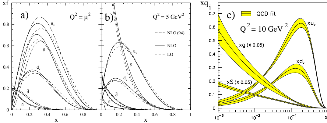
Abbildung 1.8: Partondichteverteilungen im Proton bei verschiedenen Werten von Q^2 . Abbildung a) zeigt die in [Glü-1991] angenommene Verteilung bei \mu = 0,45 \text{ GeV}^2 , aus der durch die DGLAP-Gleichungen die Dichteverteilungen bei höheren Q^2 entwickelt werden können. In Abbildung b) ist die beispielhaft für Q^2 = 5 \text{ GeV}^2 gezeigt [Glü-1998]. Experimentell können die Partondichten aus einer Parameteranpassung an HERA-Meßdaten extrahiert werden (Abbildung c) [Bot-2000].
