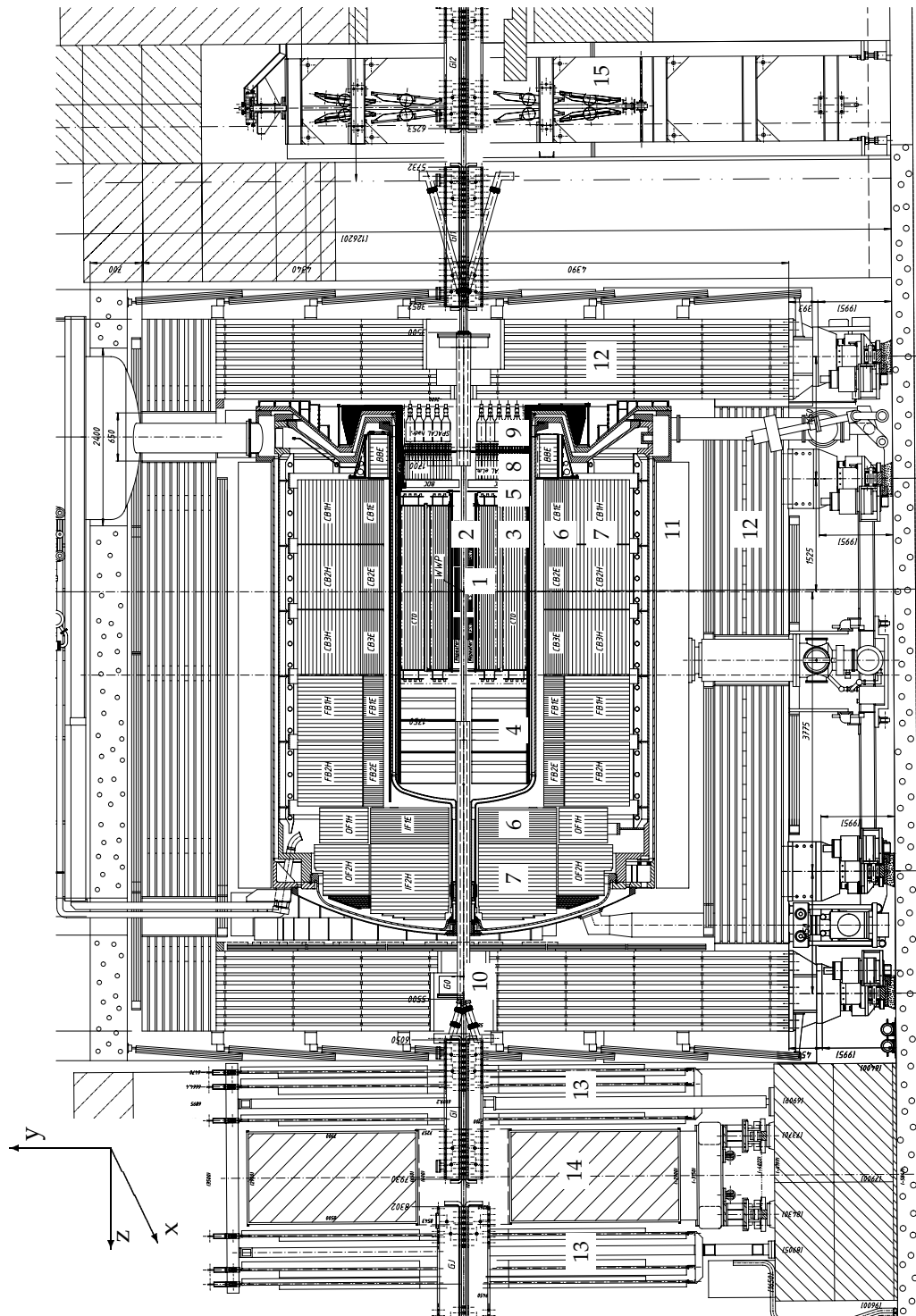
Abbildung 2.1: Längsschnitt durch den H1-Detektor für HERA-II. [Abt-1997], aktualisiert.
