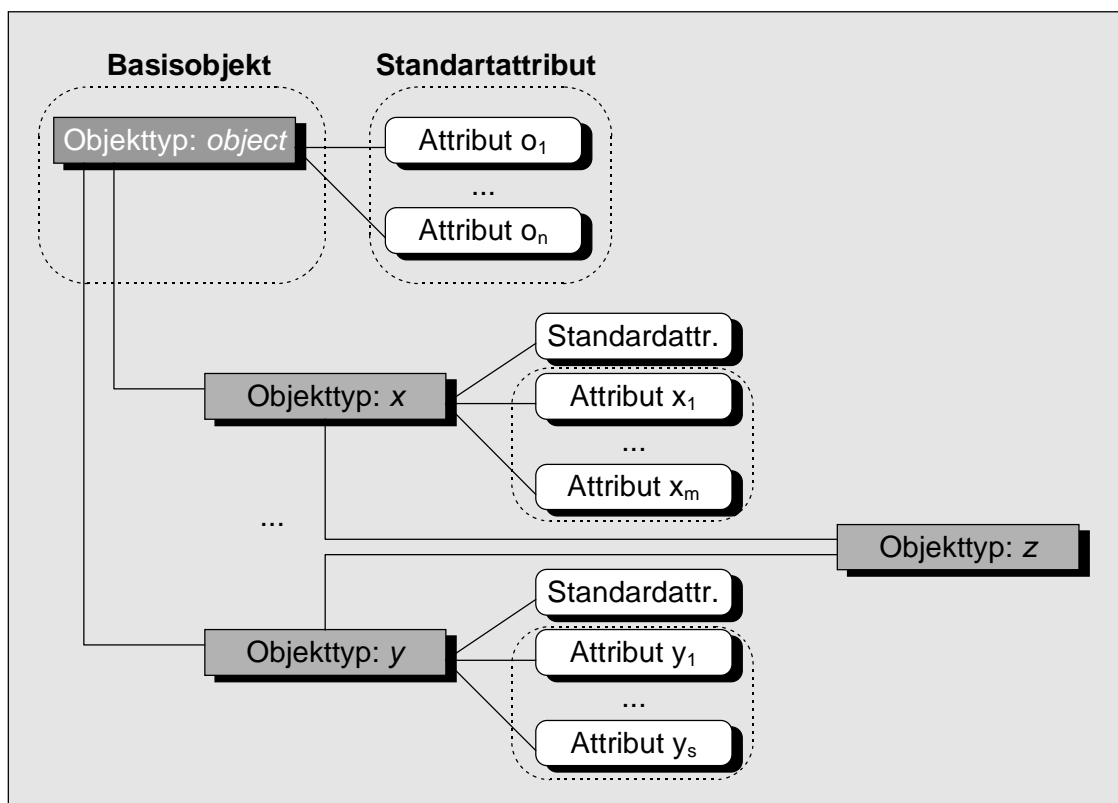
Abbildung 6: Objekthierarchie
