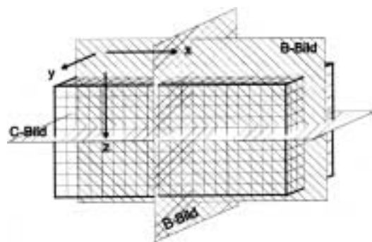
BILD 3.6: Prinzip eines C-Bildes (Quelle: Krause in [KRIEGER1998])
