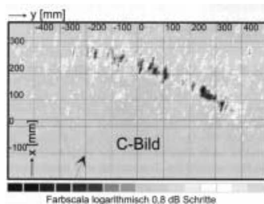
BILD 3.7: C-Bild am Probekörper BAS t 1 (Quelle: Krause in [KRIEGER1998])
