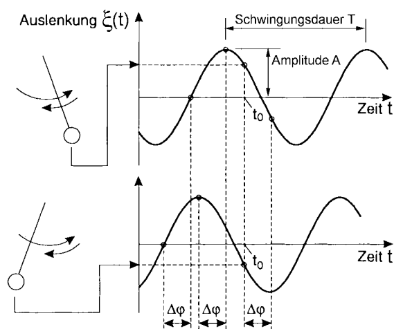
BILD 2.3: Beispiel für Amplitude und Phasendifferenz [MATTHIES1998]
