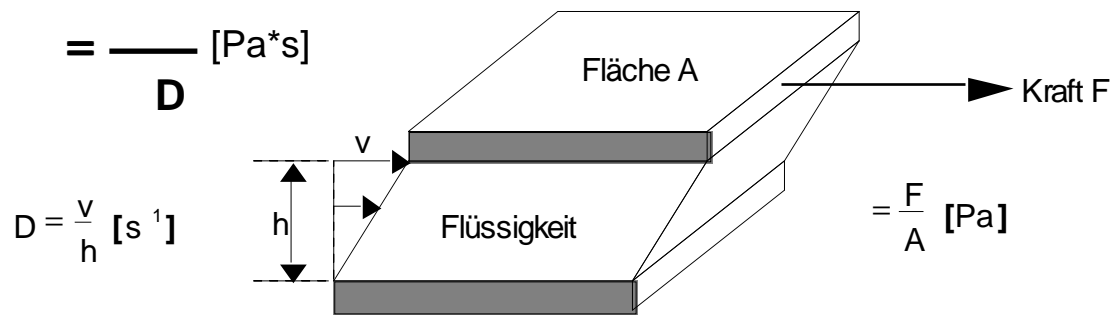
BILD 4.25: Zur Definition der dynamischen Viskosität
