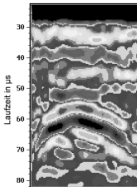
BILD 5.4: B-Bild des Hüllrohres in Probekörper BAM1 (unbewehrte Seite)
