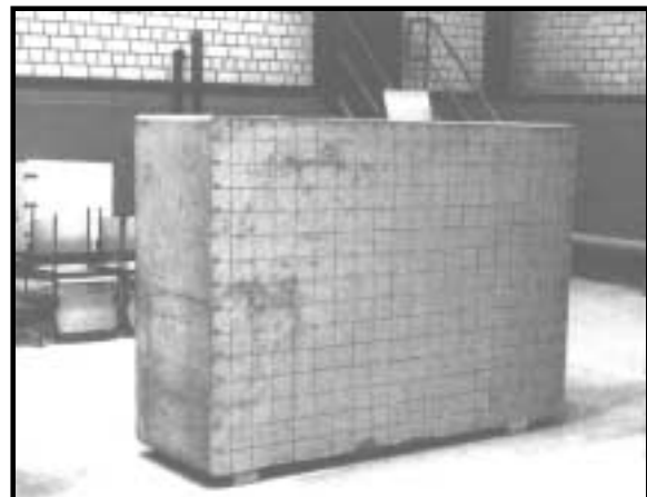
BILD 5.12: Probekörper BASt1
