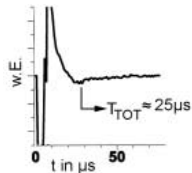
BILD 4.17: Ausschwingverhalten des Pr.kopf «4» (s.Text)
