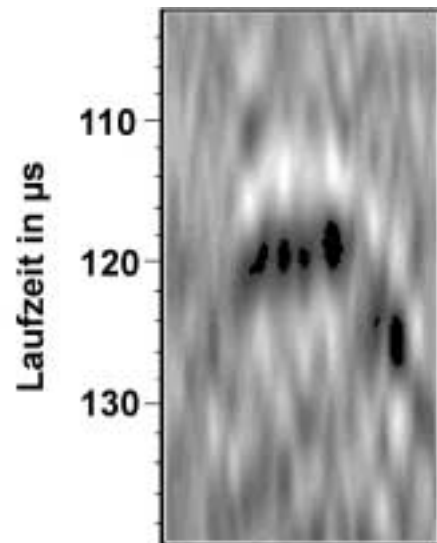
BILD 5.16: Detailansicht des Spannkanals im B-Bild
