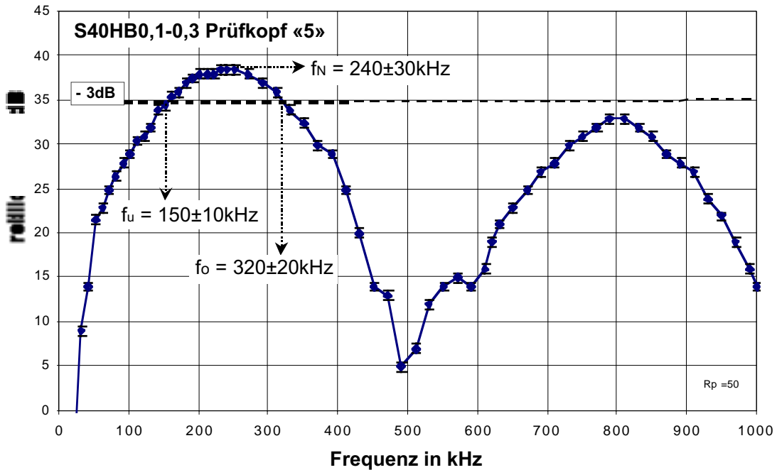
BILD 4.18: Frequenzspektrum des Prüfkopfes «5» S40HB0,1-0,3
