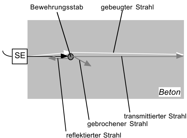
BILD 2.21: Schema: Einfluss von oberflächennaher Bewehrung
