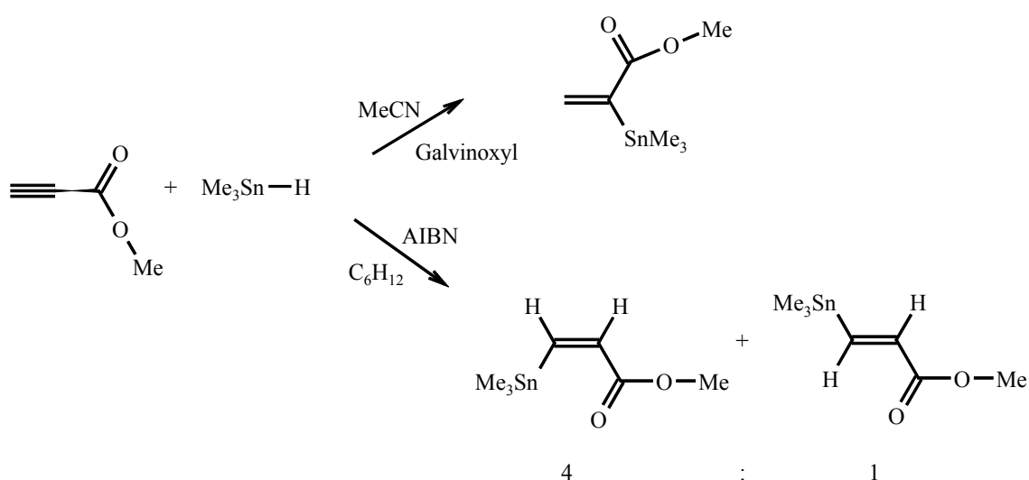
Abbildung 7: Radikalische und polare Hydrostannierung
