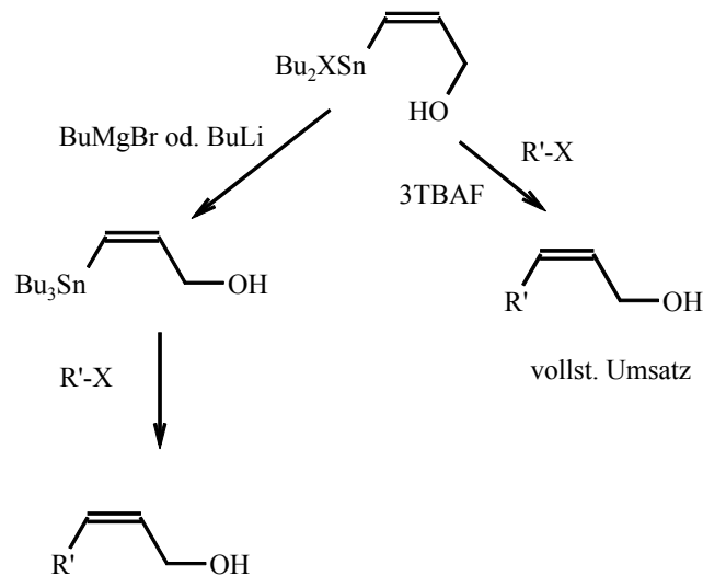
Abbildung 56: Anwendung der Hydrostannierungsprodukte in der Stille-Kupplung
