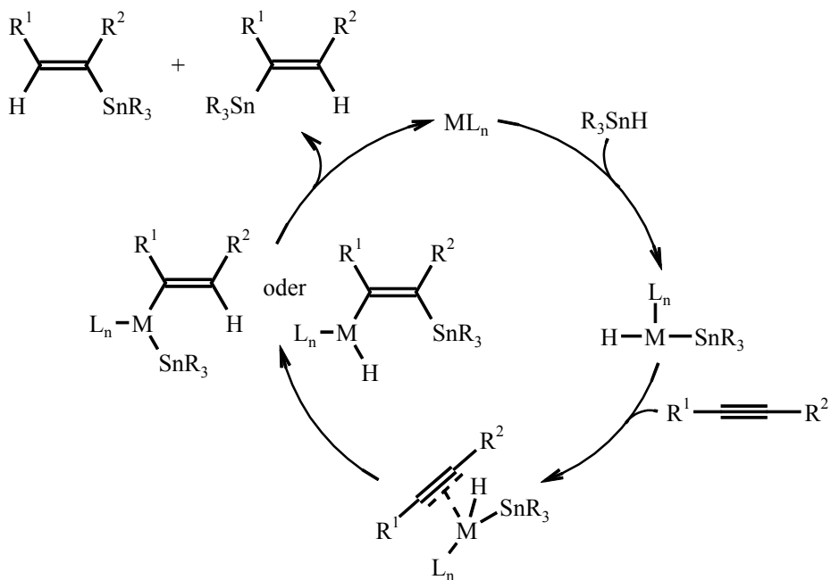
Abbildung 8: Mechanismus der Metall-katalysierten Hydrostannierung
