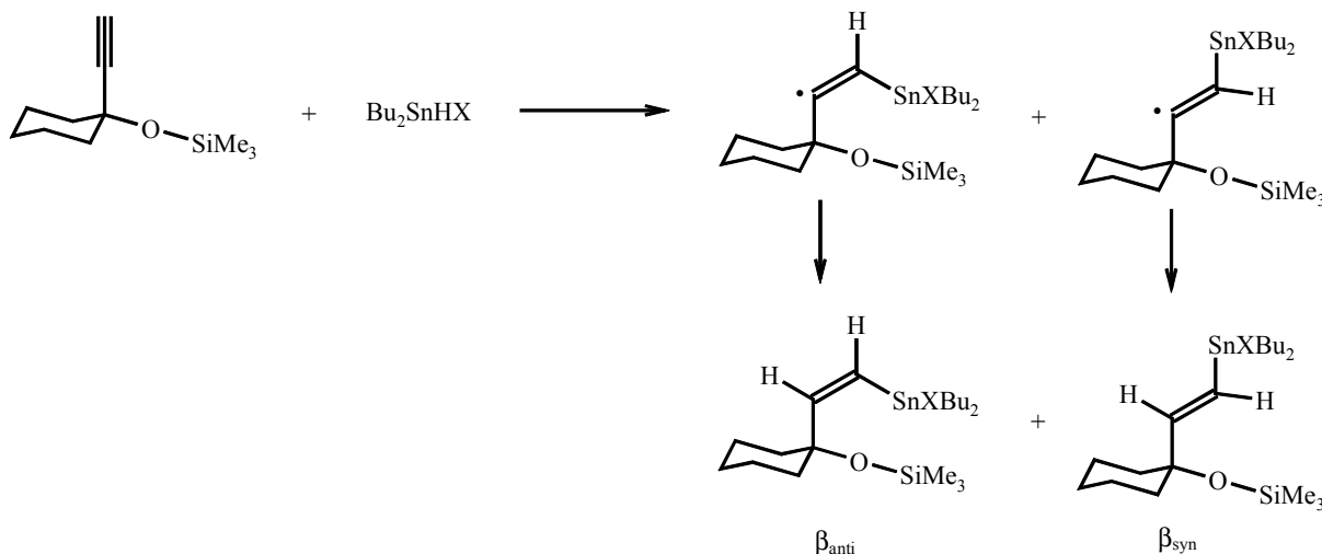
Abbildung 44: Darstellung der Verankerung des \text{O-SiMe}_3 -Gruppe in der äquatorialen Position, Ausbildung des exo -Radikals und des entsprechenden Produkts; \text{X}=\text{Cl}
