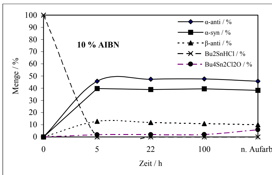
Abbildung 28: Schematische Darstellung der äquimolaren Reaktion zwischen \text{Bu}_2\text{SnHCl} und 2-Butin-1-ol bei Zugabe von 10 % AIBN (Versuch 81)
