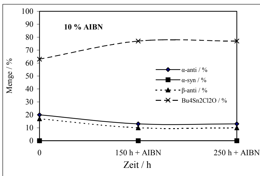
Abbildung 27: Schematische Darstellung der versuchten Isomerisierung von Z-2-Dibutylchlorostannyl-2-buten-1-ol ( \alpha_{anti} )
