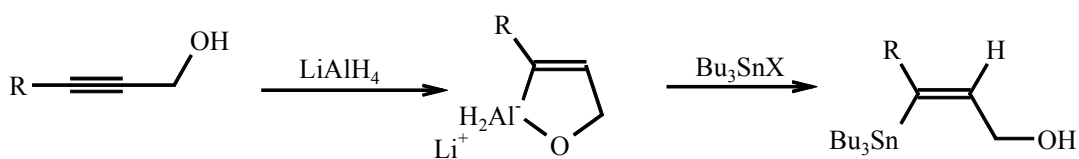
Abbildung 2: Hydroaluminierung mit anschließender Transmetallierung zum Zinn.
