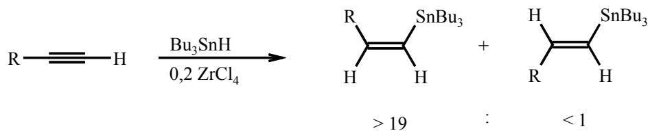
Abbildung 1: Lewisäure-katalysierte Hydrostannierung von Alkinen [1].
