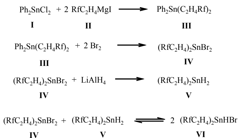
Abbildung 59: Geplante Synthese von Bis-(2-(perfluorhexyl)ethyl)zinnhydridbromid.
