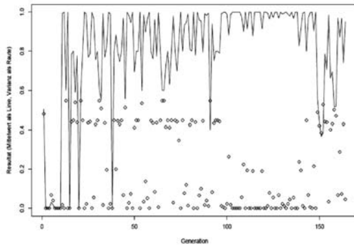
Abbildung 6.22: Der Plot zeigt das durchschnittliche Ergebnis von fünf Spielen des besten Individuums gegen einen MiniMax-Algorithmus der Tiefe 1. Die Raute geben die Varianz der Ergebnisse an. Die Kurve gibt an, ob das Individuum gewonnen (1,0) oder verloren (0,0) hat.
