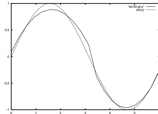
Abbildung 4.38: In dieser Graphik sieht man das Ergebnis der Evolution nach 30 Generationen, nun ist auch die zweite Hälfte der Funktion approximiert worden.
