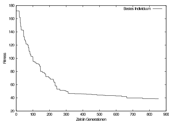
Abbildung 6.4: Bewertung Material mit einer Population von 1000 Individuen.
