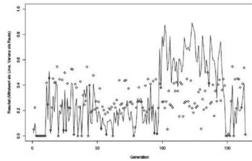
Abbildung 6.23: Der Plot zeigt das durchschnittliche Ergebnis von fünf Spielen des besten Individuums gegen einen MiniMax-Algorithmus der Tiefe 2. Die Raute geben die Varianz der Ergebnisse an. Die Kurve gibt an, ob, das Individuum gewonnen (1,0) oder verloren (0,0) hat.
