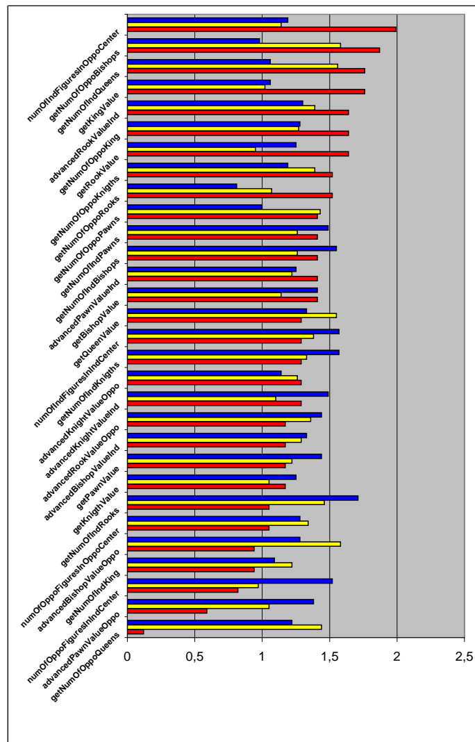
Abbildung 6.31: Der Plot zeigt ein Histogramm aller genutzten Terminalfunktionen für das Stellungsmodul. Die gelben Balken des Diagramms stellen die Evolutionsläufe der weißen Individuen mit einem Knotenlimit von 100.000 dar, die blauen die der schwarzen Individuen und die roten die mit einem Knotenlimit von 250.000, nach diesen sind Balken auch fallend sortiert.
