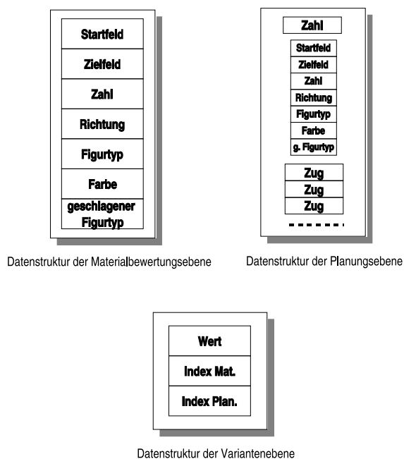
Abbildung 5.2: Die Datenstrukturen der einzelnen Ebenen des GP Systems.
