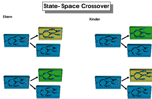
Abbildung 4.11: Die Crossoveroperation auf der Ebene des State-Space Individuums. Da das Individuum aus drei Substrukturen besteht, kann auf dieser Ebene des Crossovers nur die gesamte Substruktur getauscht werden.
