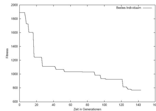
Abbildung 6.13: Materialbewertung Defensive mit einer Population von 1000 Individuen und eingeschränkter Funktionsmenge
