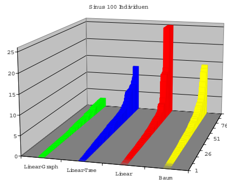
Abbildung 4.28: Die Fitness des besten Individuums in der letzten Generation von allen Strukturen. Für das Sinus Problem mit 100 Individuen.
