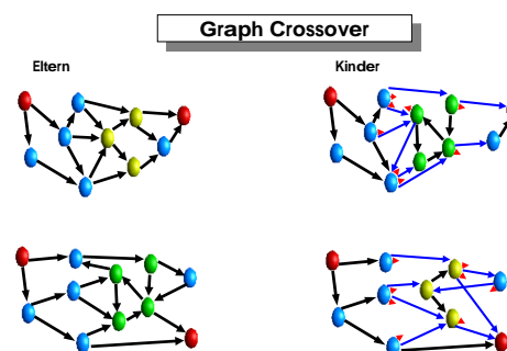
Abbildung 3.5: Graphbasiertes Crossover.
