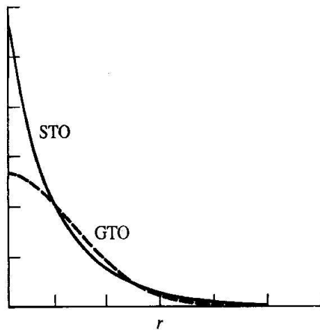
Abbildung 2.1: S later- T ype- O rbital (STO) und G auss- T ype- O rbital (GTO) im Vergleich[1]
