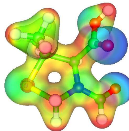
Abbildung 3.16: Elektronendichteverteilung 5-Ring Produkt
