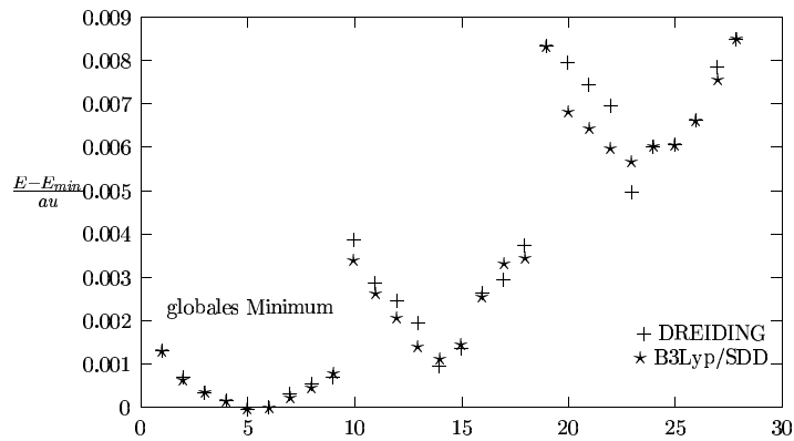
Abbildung 3.25: Vergleich der Minima von DREIDING mit B3Lyp/SDD
