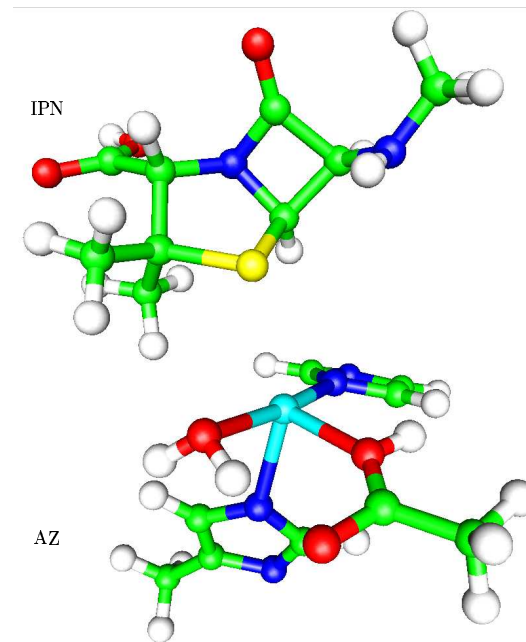
Abbildung 3.18: AZ mit IPN
