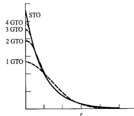
Abbildung 2.2: Linearkombinationen mehrerer GTO[1]
