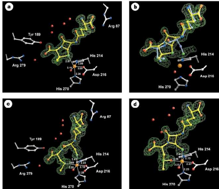
Abbildung 3.2: Röntgenstrukturen des aktiven Zentrums von INPS
