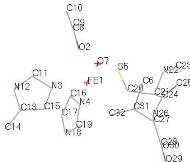
Abbildung 3.11: Katalytisches Zentrum, Atomnummerierung
