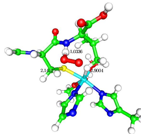
Abbildung 3.23: Sauerstoffanlagerung, Dreiding, Abstände in Å
