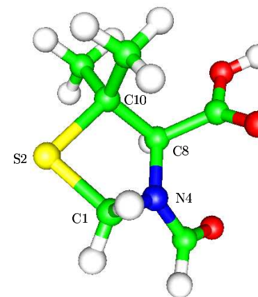
Abbildung 3.14: 5-Ring Produkt mit Atomnummerierung
