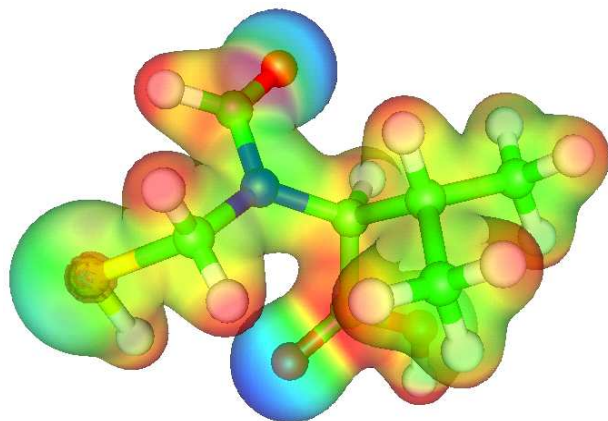
Abbildung 3.15: Elektronendichteverteilung im 5-Ring Edukt
