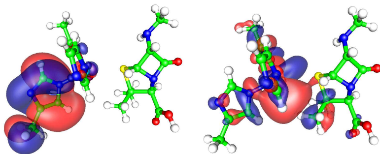
Abbildung 3.19: HOMO (AZ mit IPN)
