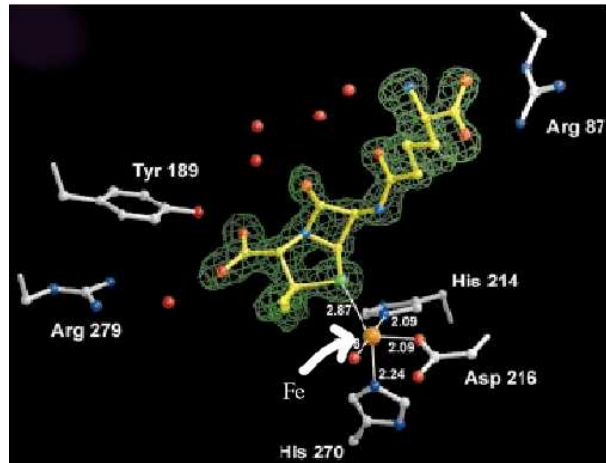
Abbildung 3.5: Ausschnitt des AZ mit IPN
