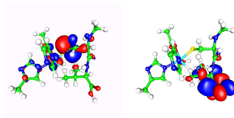
Abbildung 3.21: HOMO (AZ mit ACV)
