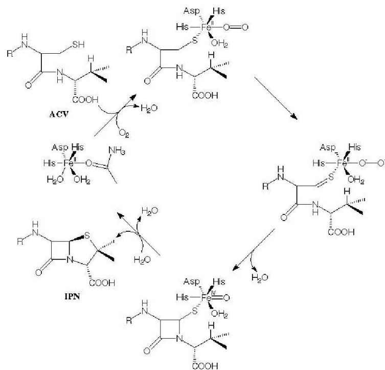
Abbildung 3.4: Postulierter Reaktionsmechanismus der IPN-Synthese
