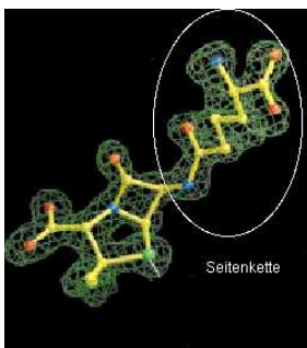
Abbildung 3.7: Darstellung der Seitenkette
