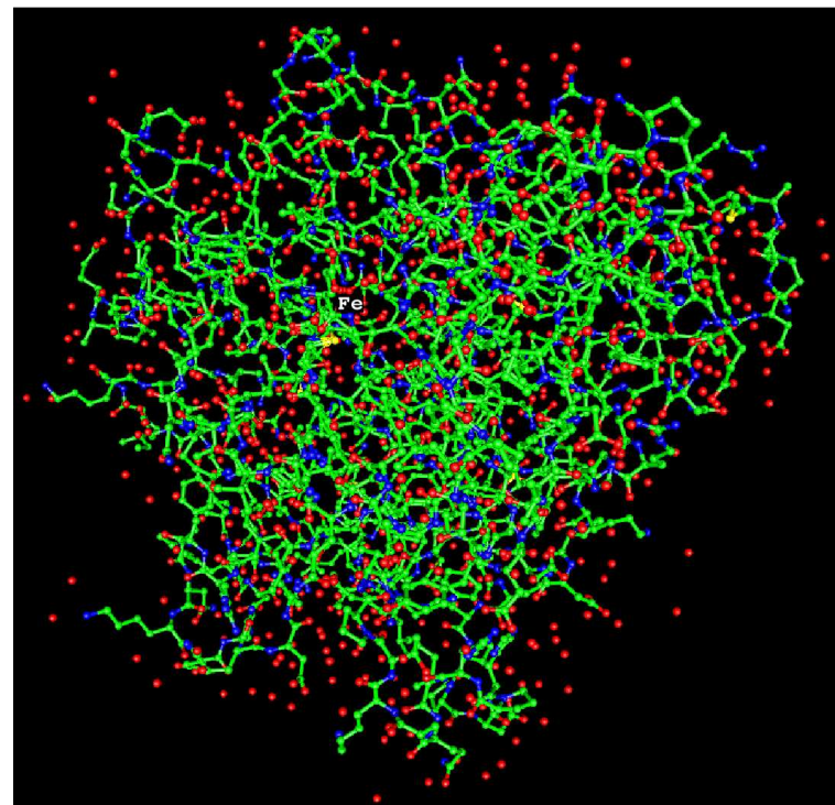
Abbildung 3.1: Röntgenstruktur der IPN[2]
