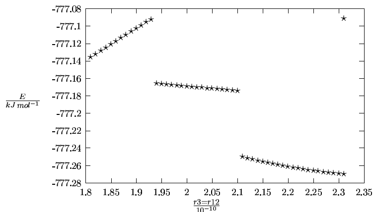
Abbildung 3.13: Ausschnitt der 4-Ringbildung aus Abbildung 3.26, \frac{1}{100} Å-Schritte
