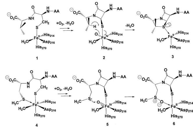
Abbildung 3.3: Mechanismus
