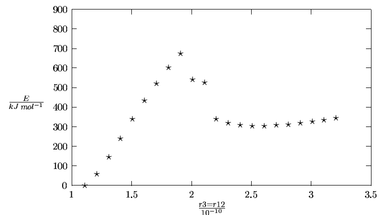
Abbildung 3.12: CD der 4-Ringbildung, Auftragung der Energie gegen den Abstand der Wasserstoffatome
