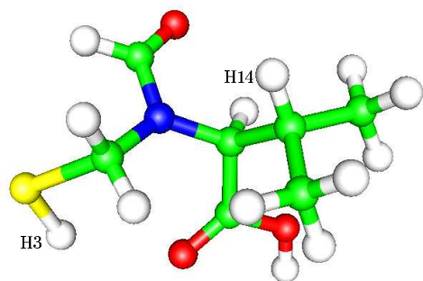
Abbildung 3.17: 5-Ring Edukt, Atomnummerierung
