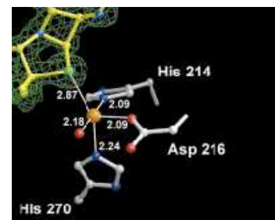
Abbildung 3.8: Katalytisches Zentrum
