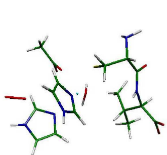
Abbildung 3.27: Lokales Minimum
