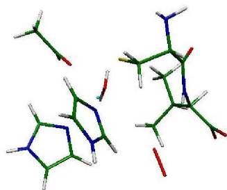
Abbildung 3.28: Globales Minimum
