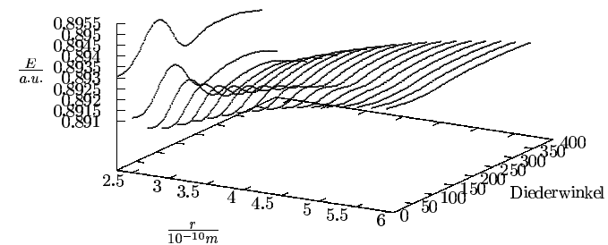
Abbildung 3.26: Hyperfläche mit 10800 Datenpunkten
