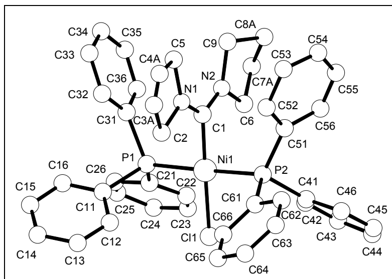
Abb. 25: Kristallstruktur des acyclischen Diaminocarben-Ni-Komplexes 261 .
