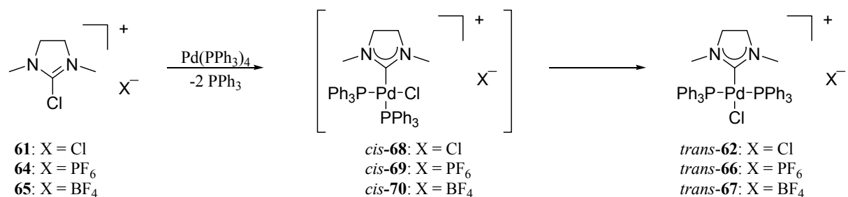
Scheme 37: Oxidative Addition und anschließende Isomerisierung zum trans -Komplex.
