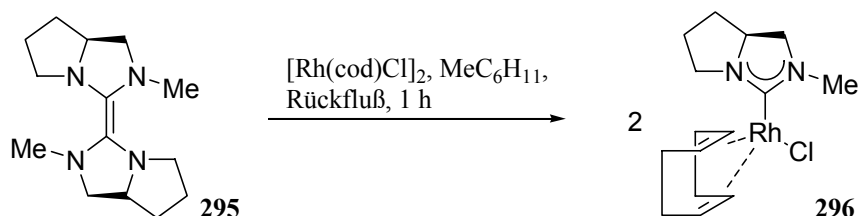
Schema 134: Darstellung des NHC-Rh-Komplexes 296 . [73, 256, 257]
