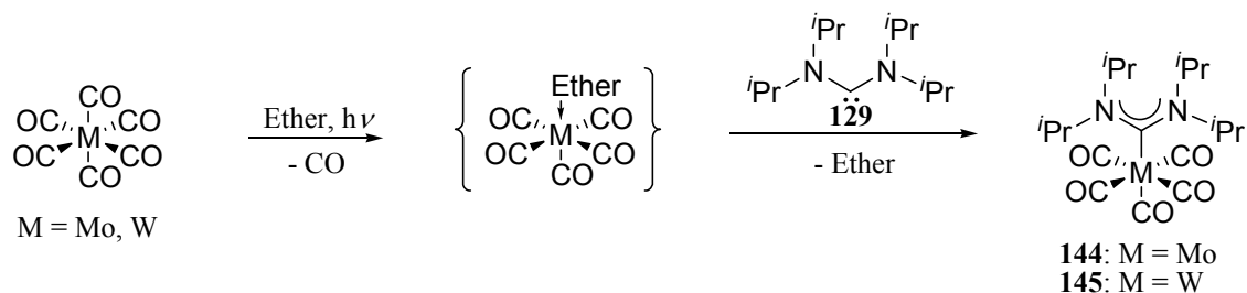
Schema 68: Reaktion von Bis(diisopropyl)-aminocarben ( 129 ) mit \text{Mo}(\text{CO})_6 und \text{W}(\text{CO})_6 . [153]
