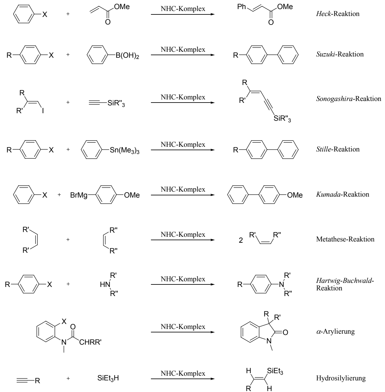
Schema 18: Eine Auswahl von NHC-Komplexen katalysierten Reaktionen.
