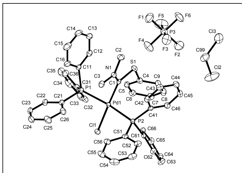
Abb. 21: Kristallstruktur des Aminothiophenoxycarben-Pd-Komplex 243 .
