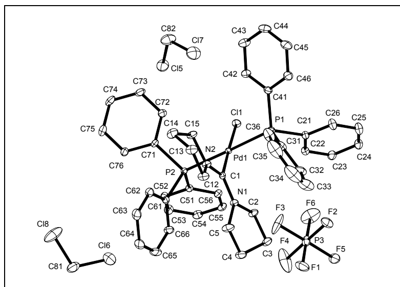
Abb. 10: Kristallstruktur des acyclischen Pd-Diaminocarbon-Komplexes 154a .
