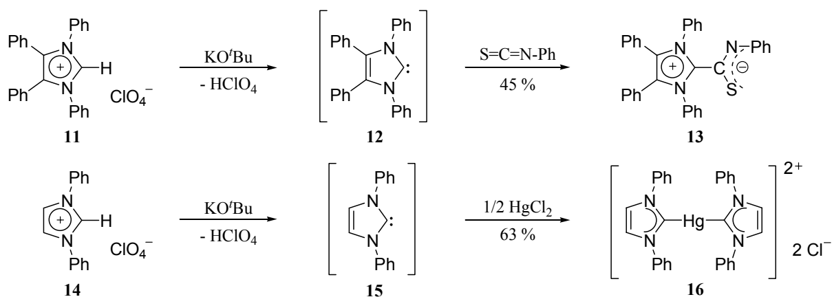
Schema 5: Darstellung von NHC als Intermediat durch Deprotonierung mit \text{KO}^t\text{Bu} . [16, 23]
