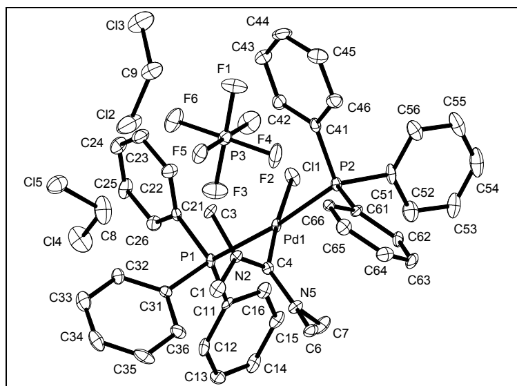
Abb. 8: Kristallstruktur des acyclischen Pd-Diaminocarbon-Komplexes 152 .
