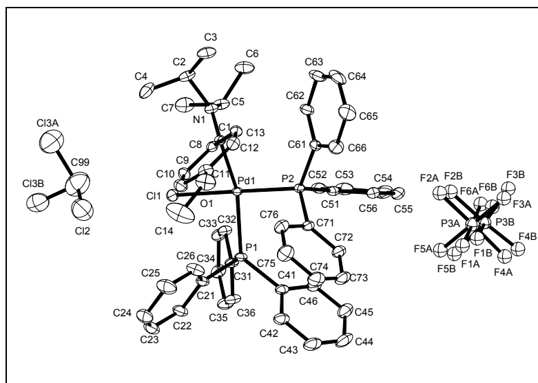
Abb. 15: Kristallstruktur des Aminoarylcarben-Pd-Komplexes 199 .
