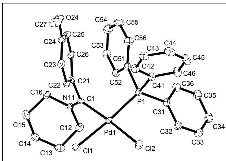
Abb. 16: Kristallstruktur des Aminoarylcarben-Pd-Komplexes 203 .
