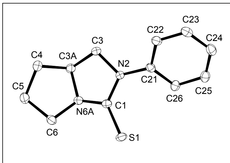
Abb. 28: Kristallstruktur des Thioharnstoffderivates 85 .
