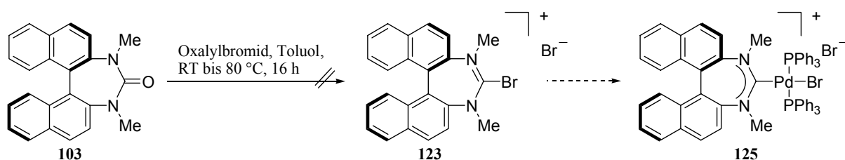
Schema 57: Versuchte Synthese des Imidazoliumbromids 123 .
