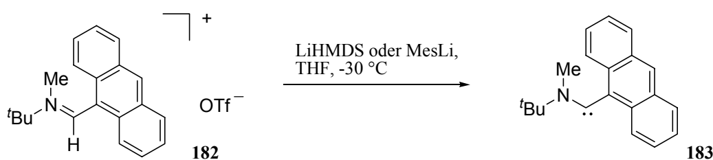
Schema 85: Darstellung von Aminoarylcarben 183 . [195]
