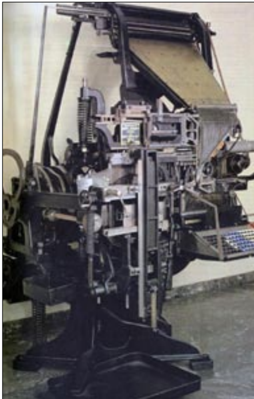
Abb. 28: Linotype, Modell 1, die erste funktionierende Zeilensetzmaschine der Welt, konstruiert und hergestellt in den USA.
