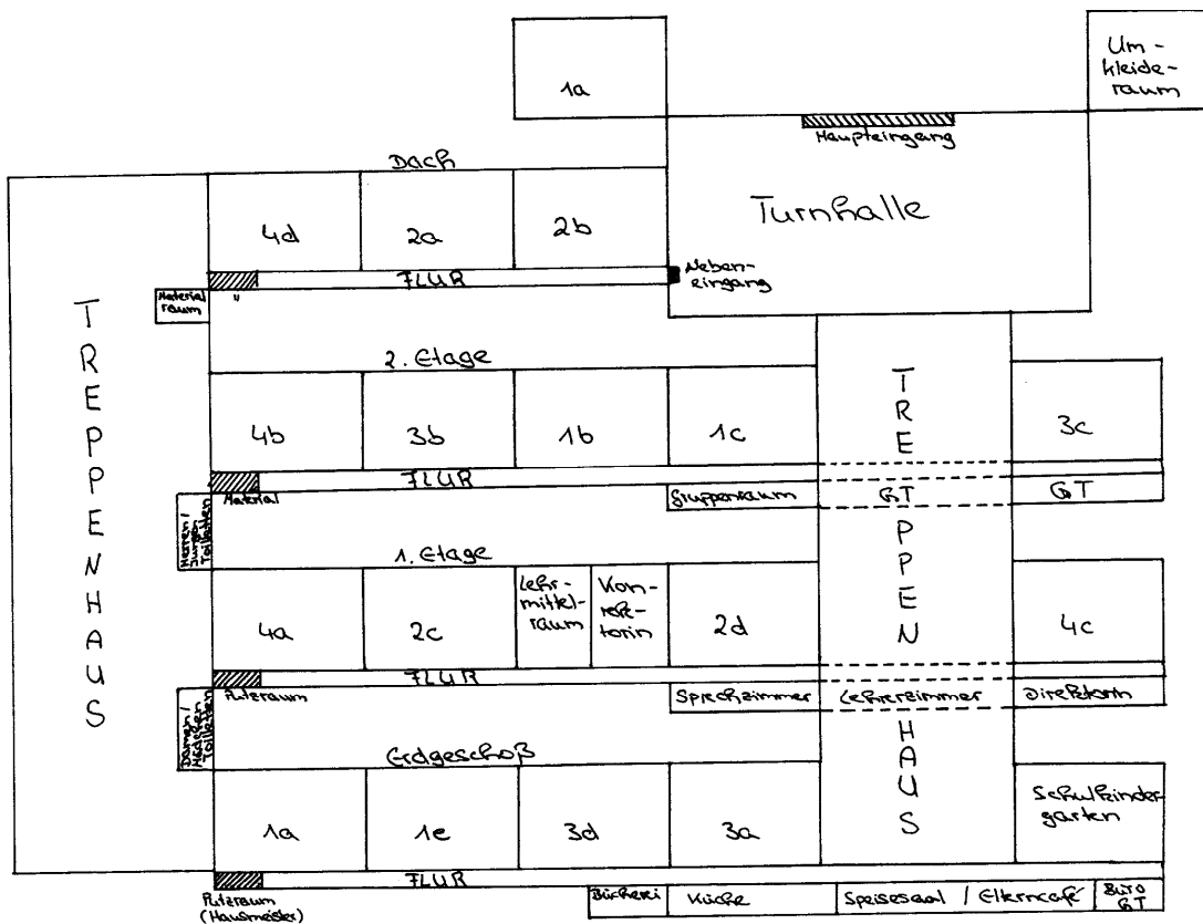
Abb. 33: Handskizze – Raumplan eines Schulgebäudes
